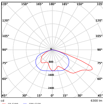
LEDPostTop-P 50W-AS
