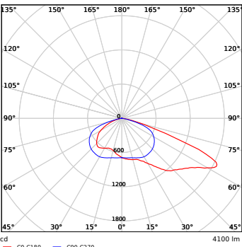
LEDPostTop-P 33W-AS
